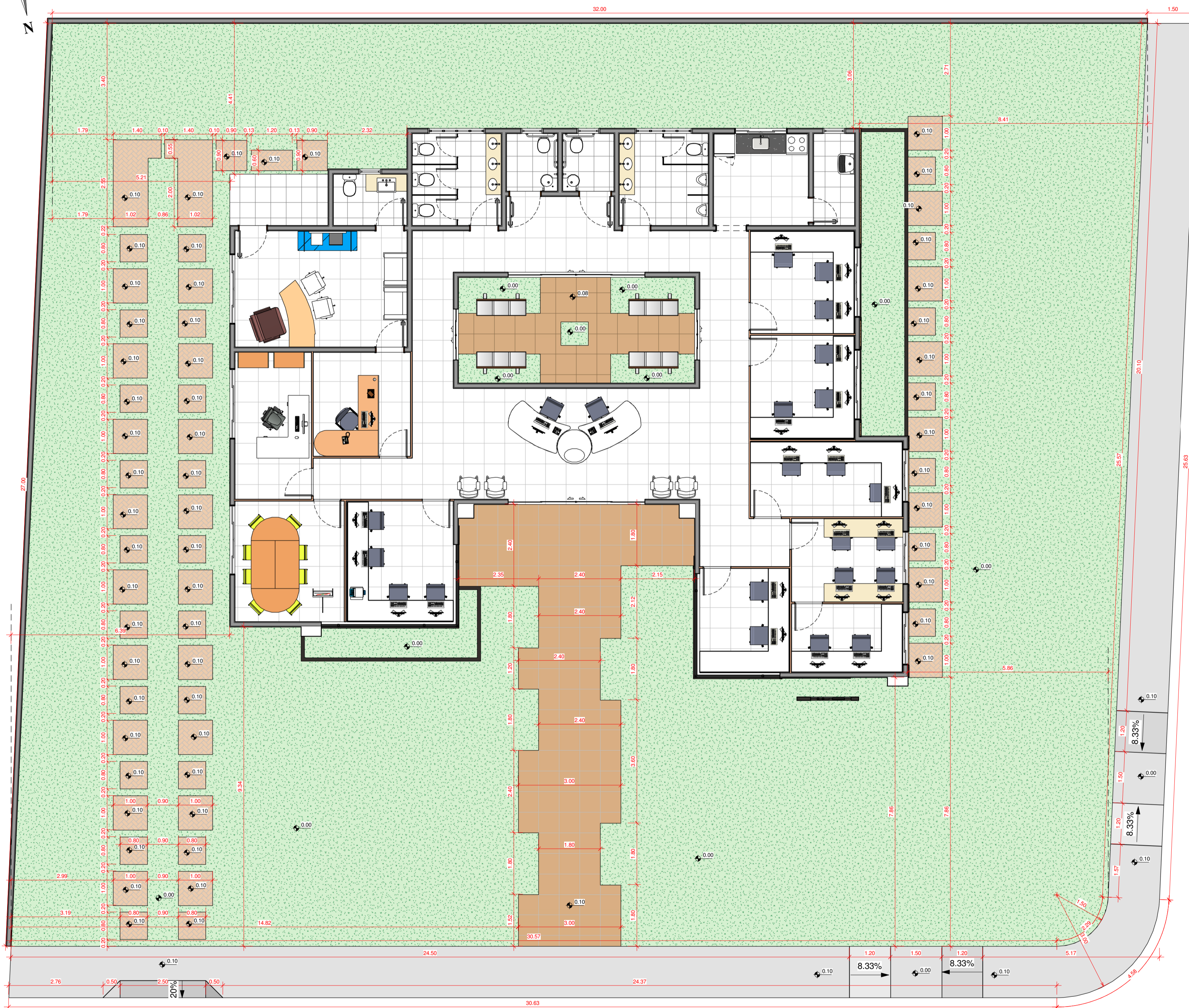
1 IMPLANTAÇÃO 1 : 75
