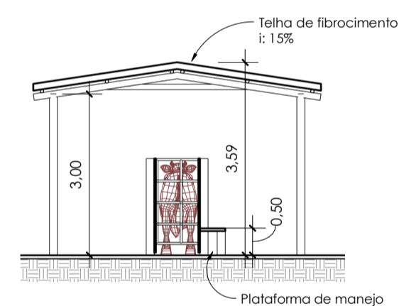
3 Corte AA - Cobertura Brete de Solta e Chegada 1:100
