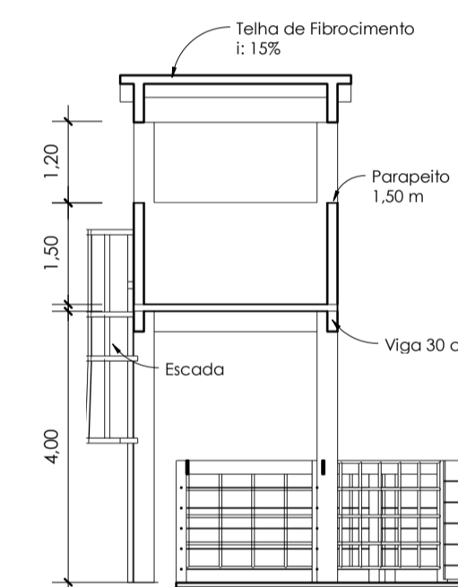
6 Corte DD - Cabine Locutor 1:100
