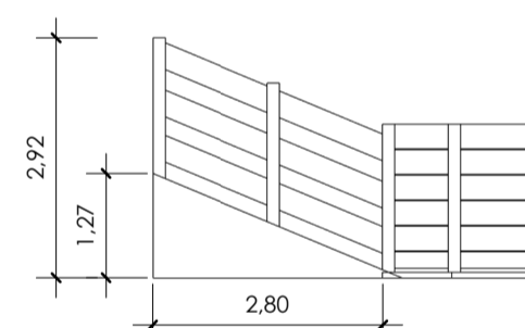
4 Corte BB - Brete de Carga 1:100
