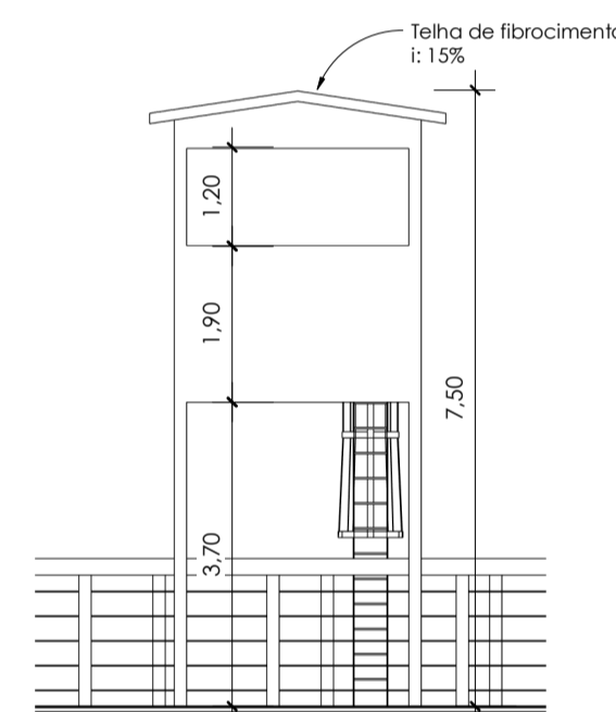
5 Corte CC - Cabine Locutor 1:100
